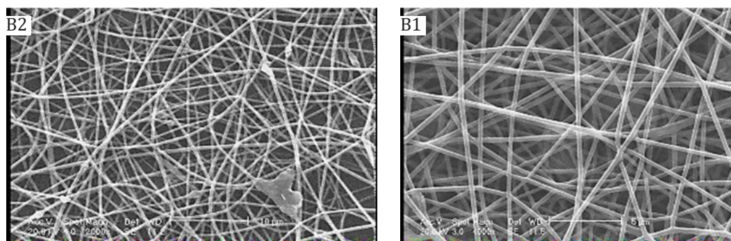
شکل ۸: تصاویر میکروسکوپ الکترونی پویشی از نمونه های B1، B2 Fig 8: SEM images of B1, B2 samples
