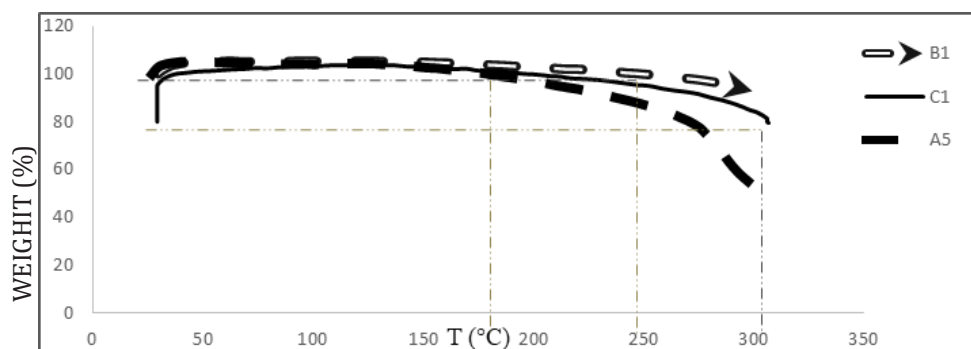
شکل ۱۲: الگوی TGA از الیاف نمونه های A5، B1، C1 Fig 12: TGA traces of C1, B1 and A1 fibers
