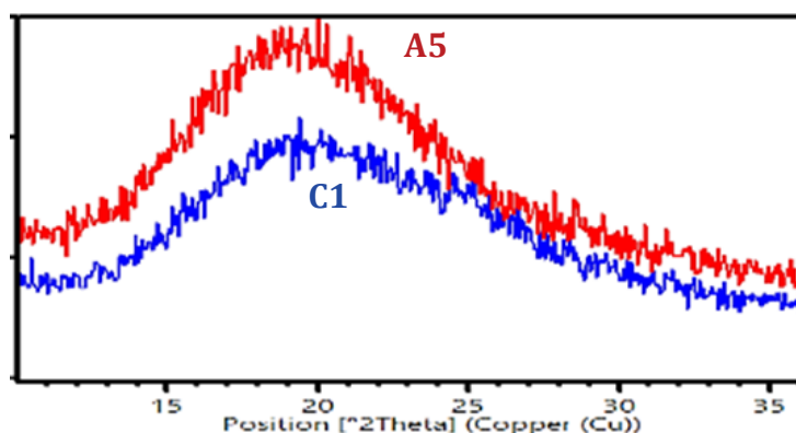
شکل ۶: مقایسه نتایج پراش پرتوی ایکس از نانوالیاف C1: PVA/۰.۴gr G تحت فراصوت میله‌ای و A5: PVA Fig 6: Comparison of XRD patterns of nanofiber C1: PVA/0.4gr graphite treated by ultrasonic probe and A5: PVA
