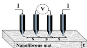
شکل ۱: طرح واره دستگاه چهار کاوند نقطه‌ای برای اندازه‌گیری رسانایی الکتریکی [۱۸]
