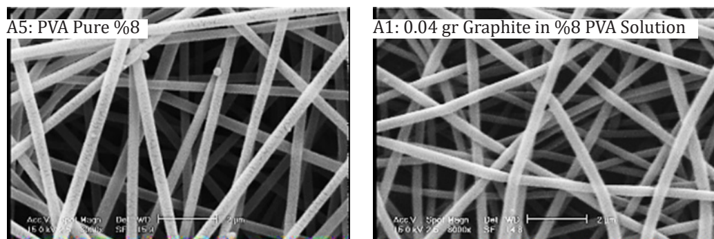
شکل ۷: تصاویر میکروسکوپ الکترونی پویشی الیاف الکتروریسی شده Fig 7: SEM images of A1, A5 electrospun fibers
