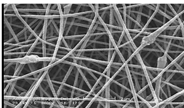
شکل ۱۰: تصویر میکروسکوپ الکترونی پوششی الیاف الکترونیسی شده C۱ (تحت فراصوت میله‌ای)
