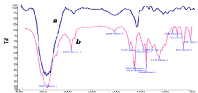
شکل ۱ طیف (a) نانواکسید گرافن، (b) نانوکامپوزیت GO/PMMA (GP2) Figure 1 FTIR spectra a) nanographene oxide, b) GO/PMMA (GP2) nanocomposite
