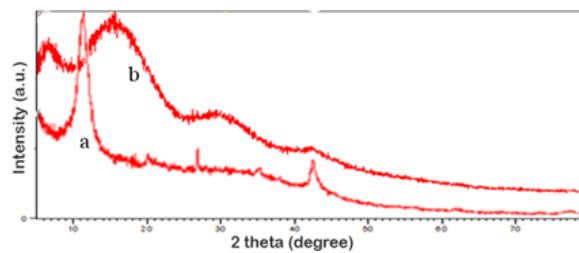
شکل ۲ طیف (XRD ، a) نانوکامپوزیت GO/PMMA (نمونه ۲) Figure 2 XRD spectra a) nanographene oxide, b) GO/PMMA (GP2) nanocomposite
