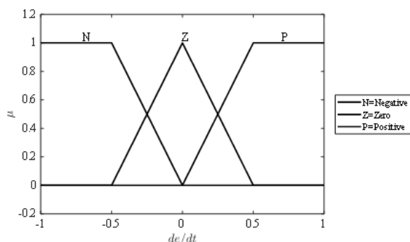
شکل ۷ توابع عضویت فازی سازی مشتق خطا Figure 7. Error derivative Fuzzification membership functions
