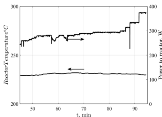
شکل ۱۴ دمای مرحله استری شدن و گرمای اعمال شده
