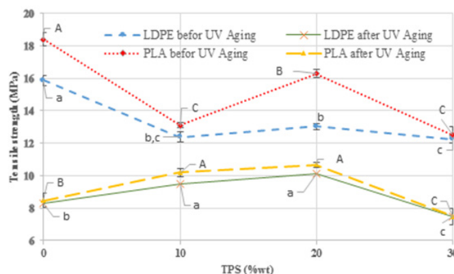
شکل ۵ مقادیر استحکام کششی در فیلم های با درصدهای مختلف نشاسته گرمانرم (حروف لاتین غیریکسان بیانگر معنی داری در سطح احتمال p < 0.05 )
