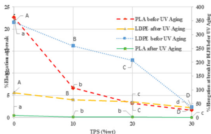
شکل ۶ تغییرات درصد ازدیاد طول در نقطه شکست در فیلم های با درصدهای مختلف نشاسته گرمانرم (حروف لاتین غیریکسان بیانگر معنی داری در سطح احتمال p < 0.05 )
