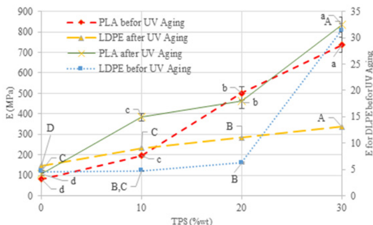
شکل ۷ تغییرات مدول کشسانی در فیلم های با درصدهای مختلف نشاسته گرمانرم (حروف لاتین غیریکسان بیانگر معنی داری در سطح احتمال p < 0.05 )
