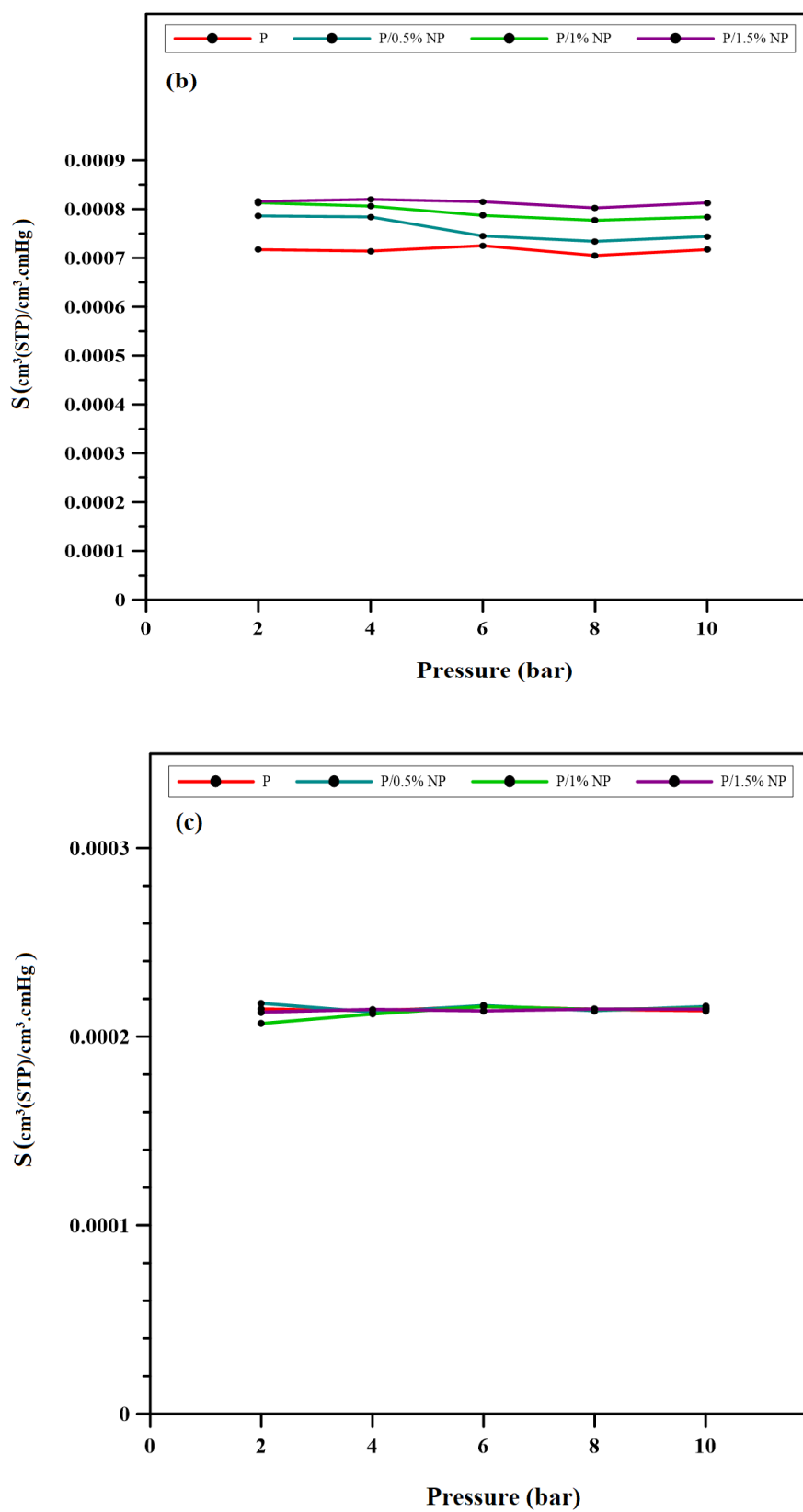
شکل ۸. اثر فشار بر ضریب حلالیت گازهای (الف) CO ۲ ، (ب) CH ۴ و (پ) N ۲ . Figure 8. The effect of pressure on solubility coefficient of (a) CO 2 , (b) CH 4 , and (c) N 2
