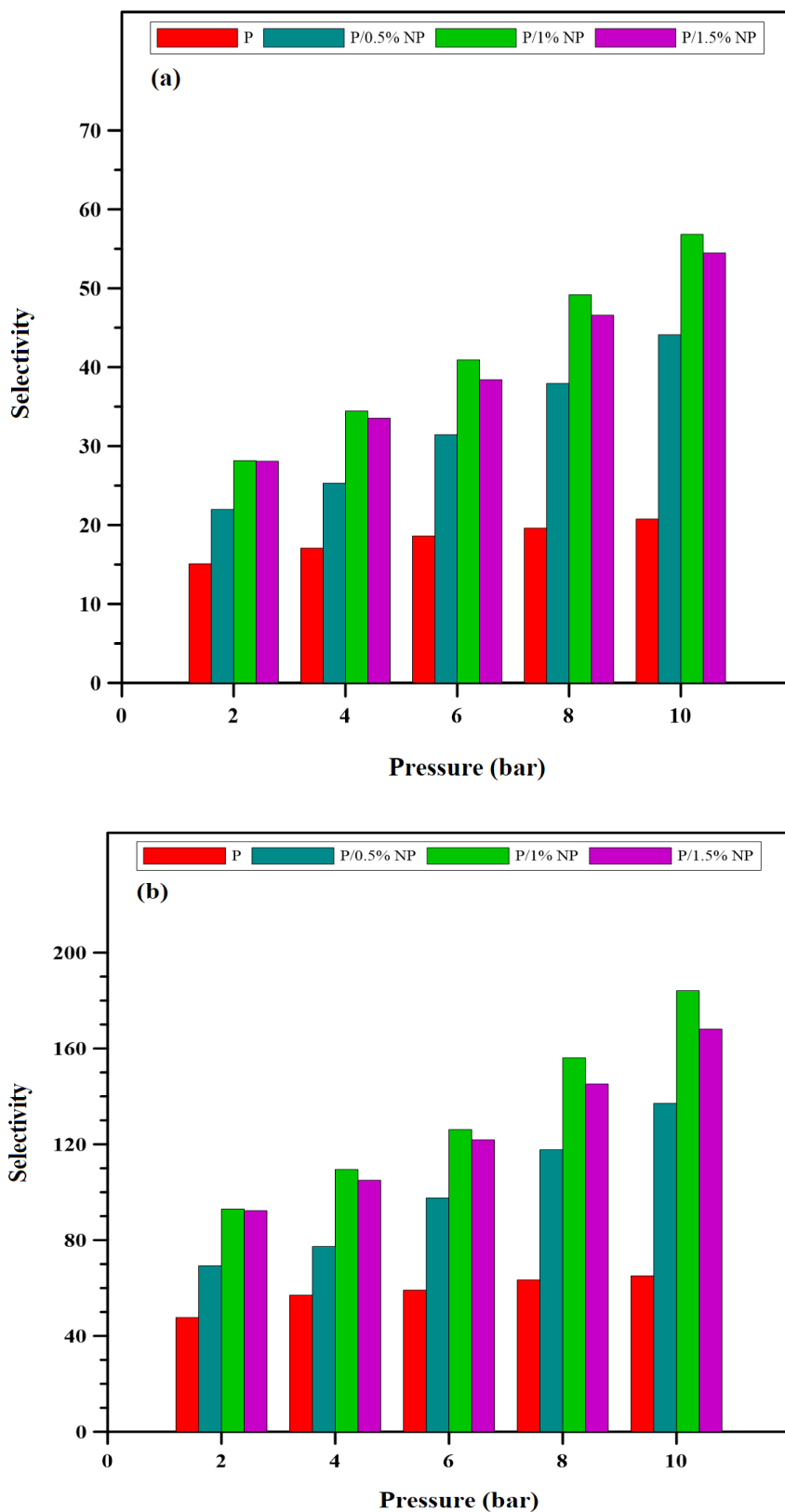
شکل ۱۰. اثر فشار بر گزینش پذیری (الف) \text{CO}_2/\text{CH}_4 و (ب) \text{CO}_2/\text{N}_2 Figure 10. The effect of pressure on selectivity of (a) \text{CO}_2/\text{CH}_4 and (b) \text{CO}_2/\text{N}_2
