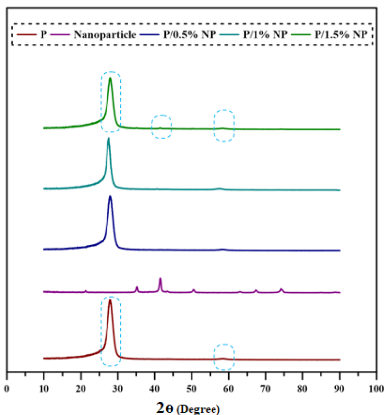
شکل ۴. نتایج مربوط به تحلیل XRD Figure 4. The results of XRD analysis
