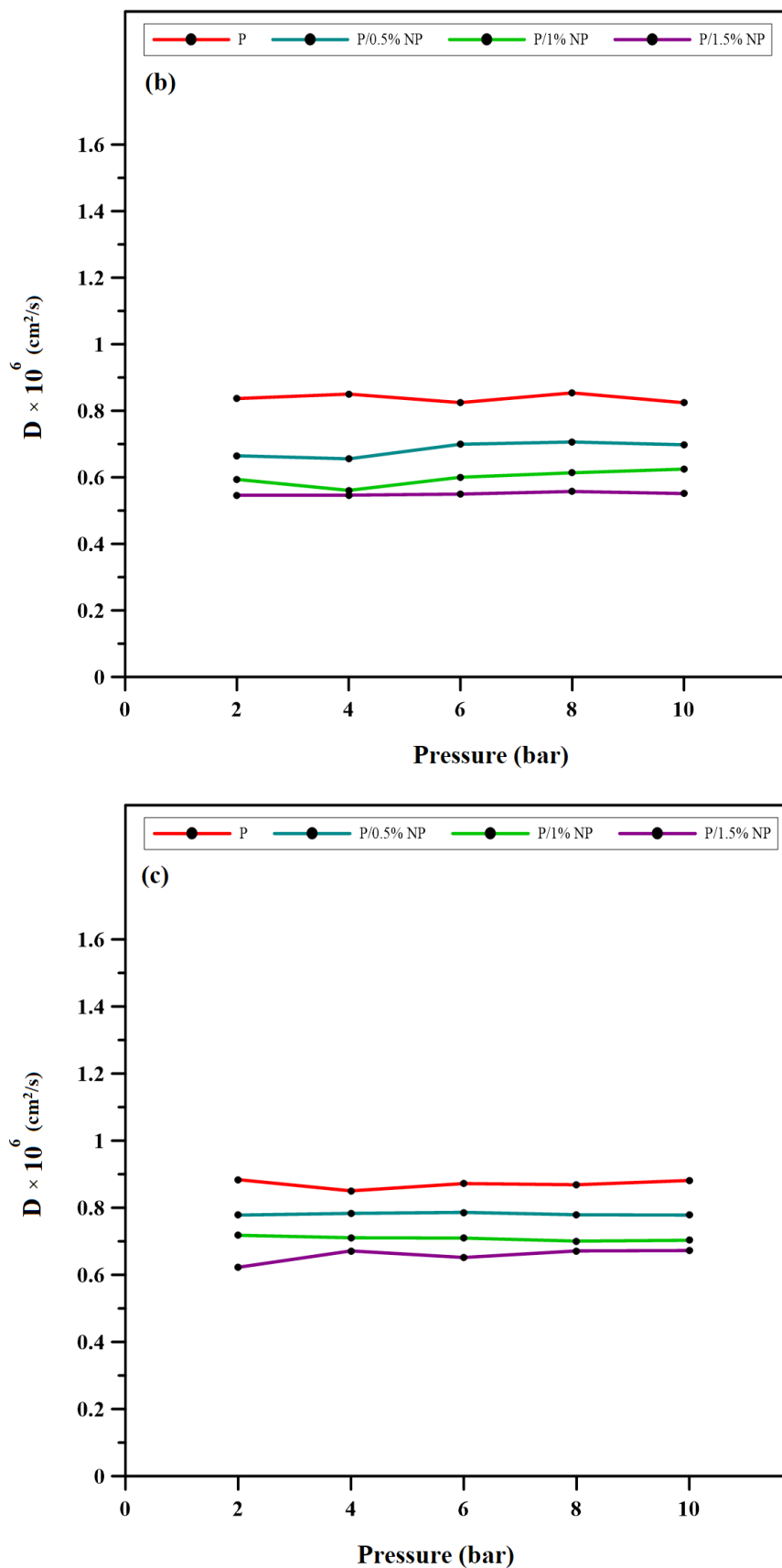
شکل ۷. اثر فشار بر ضریب نفوذ گازهای (الف) \text{CO}_2 ، (ب) \text{CH}_4 و (پ) \text{N}_2 Figure 7. The effect of pressure on diffusion coefficient of (a) \text{CO}_2 , (b) \text{CH}_4 , and (c) \text{N}_2
