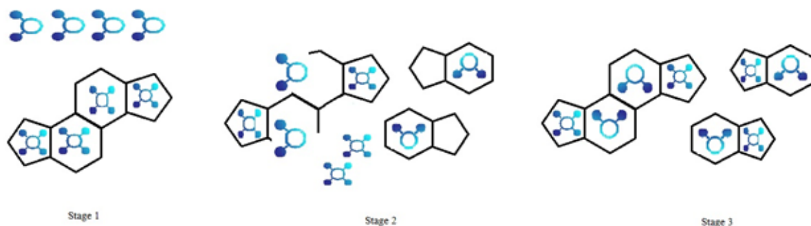
شکل ۲. سازوکار سینتیکی جایگزینی دی اکسید کربن در دوغابه ای از هیدرات متان Figure 2. The proposed mechanism for carbon dioxide replacement in a slurry of methane hydrate
