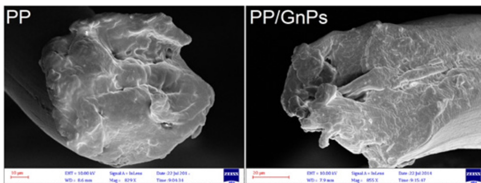
شکل ۸. تصاویر SEM سطح مقطع عرضی الیاف گسیخته PP خالص و PP/GnPs در آزمون کشش Figure 8. The cross-sectional SEM images of tensile fractured of neat PP fiber and PP/GnPs nanocomposite fiber
