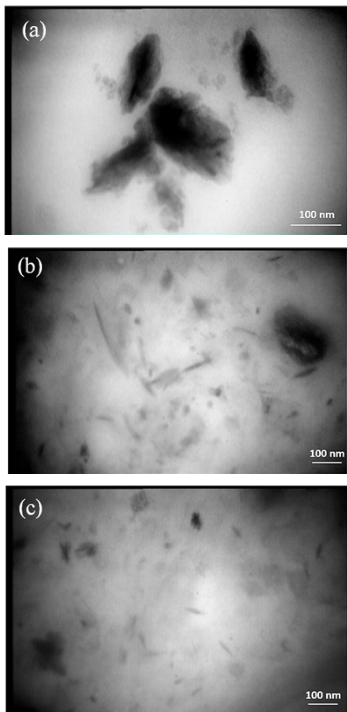
شکل ۲. تصاویر TEM از نحوه پخش و میزان تجمعات GnPs در الیاف نانوکامپوزیت PP/G0.5 و (a,b) و PP/MA/G0.5 (c) Figure 2. TEM images of GnPs dispersion state and aggregates in PP/G0.5 (a,b) and PP/MA/G0.5 nanocomposite fibers (c)
