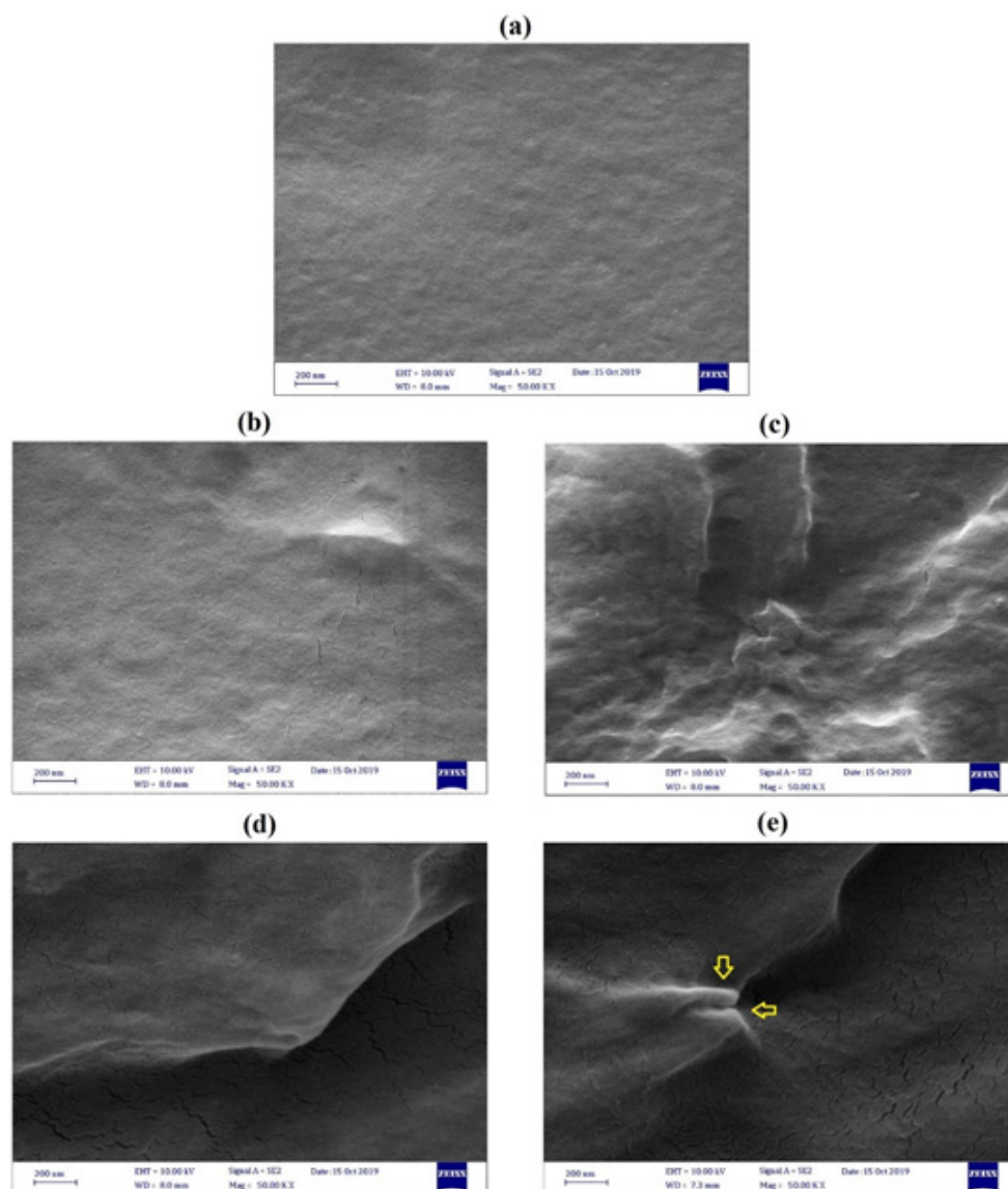
شکل ۵. تصاویر FESEM از سطح مقطع غشاهای (a) Pebax 1657، (b) Pebax/PVA حاوی ۵ درصد وزنی PVA، (c) Pebax/PVA حاوی ۱۰ درصد وزنی PVA، (d) Pebax/PVA حاوی ۱۵ درصد وزنی PVA و (e) Pebax/PVA حاوی ۲۰ درصد وزنی PVA با بزرگنمایی ۵۰ هزار برابر Figure 5. The cross-sectional FESEM images of (a) Pebax 1657, (b) Pebax/PVA 5/95, (c) Pebax/PVA 10/90, (d) Pebax/PVA 15/85, and (e) Pebax/PVA 20/80 membranes with the magnification of \times 50k
