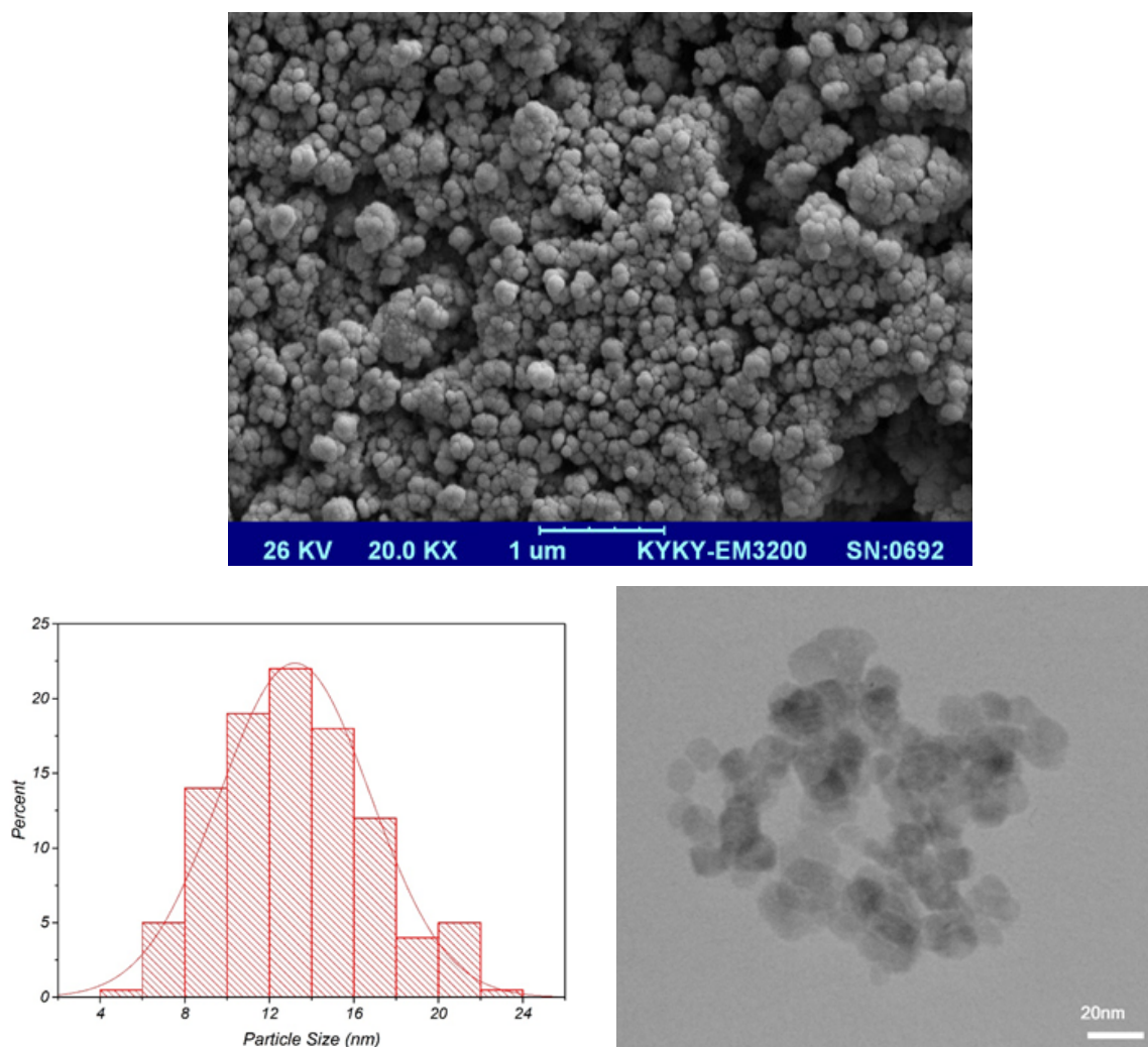
شکل ۴. (الف) تصویر SEM، (ب) تصویر TEM و (پ) نمودار توزیع اندازه ذرات اکسید ترکیبی Ce_xZr_{1-x}O_2 Figure 4. (a) SEM image, (b) TEM image, and (c) particle size distribution diagram of Ce_xZr_{1-x}O_2 mixed oxide nanoparticles
