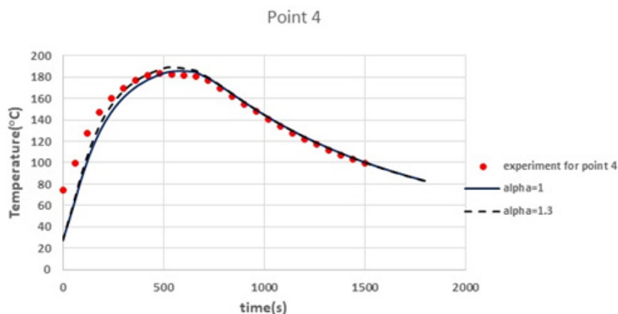
شکل ۶- تغییرات دمایی نقطه ای داخل تایر (مرز بلادر و لایه) در شرایط واقعی پخت بدست آمده از سیم گذاری و ثبت پروفایل دمایی (نقاط)، و شبیه سازی با مقادیر مختلف ضریب نفوذ حرارتی بلادر - خط \alpha=1 \times 10^{-7} و نقطه چین \alpha=1,3 \times 10^{-7}
