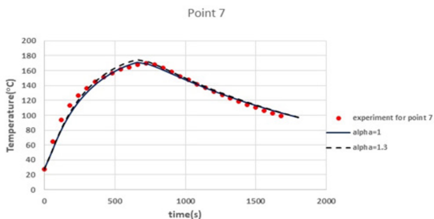
شکل ۷- تغییرات دمایی نقطه ای داخل تایر (مرکز رویه) در شرایط واقعی پخت بدست آمده از سیم گذاری و ثبت پروفایل دمایی (نقاط)، و شبیه سازی با مقادیر مختلف ضریب نفوذ حرارتی بلادر - خط \alpha=1 \times 10^{-7} و نقطه چین \alpha=1,3 \times 10^{-7}
