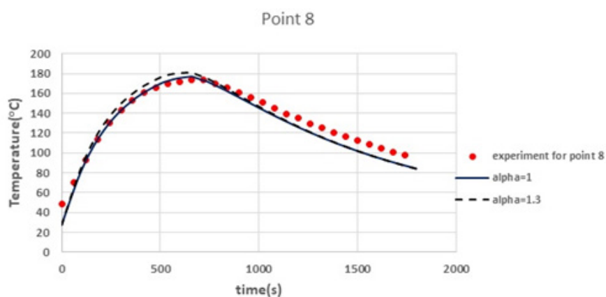
شکل ۸- تغییرات دمایی نقطه ای داخل تایر (داخل لایه) در شرایط واقعی پخت بدست آمده از سیم گذاری و ثبت پروفایل دمایی (نقاط)، و شبیه سازی با مقادیر مختلف ضریب نفوذ حرارتی بلادر (خط \alpha=1 \times 10^{-7} و نقطه چین \alpha=1,3 \times 10^{-7} )
