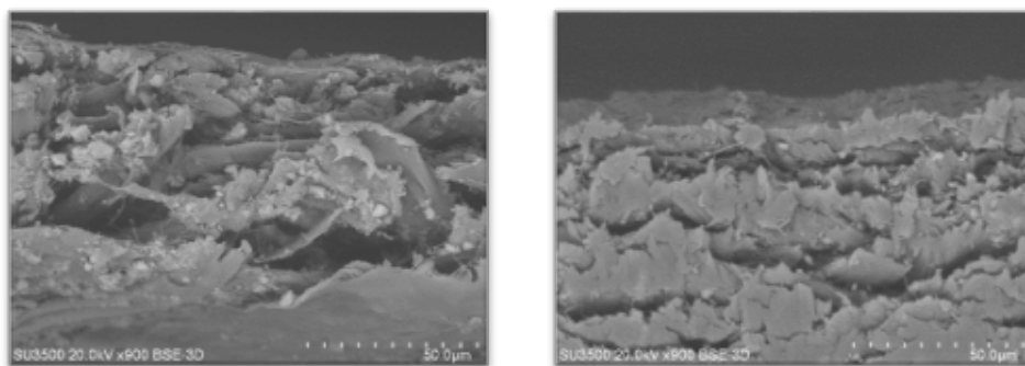
شکل ۴ تصاویر SEM سطح کاغذها در بزرگ نمایی ۲۰۰۰ از الف) نمونه کاغذ شاهد، ب) نمونه حاوی نانوهیدروژل کیتوسان-آکریلیک اسید. Fig. 4. SEM images (2000 X) of uncoated paper surface (a) and paper surface coated with chitosan/ acrylic acid nano hydrogel.
