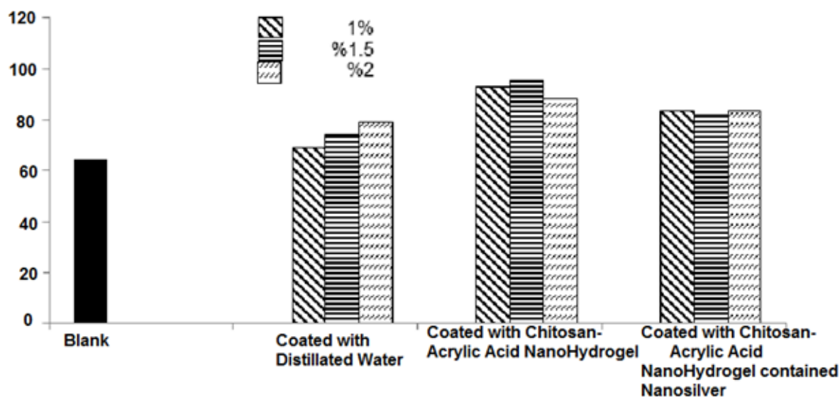
شکل ۵. مقایسه درصد جذب آب کاغذهای شاهد و اندودشده با نانوهیدروژل های مختلف. Fig. 5. Water absorption of paper coated with different nano hydrogels.
