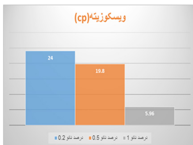
شکل ۹ نمودار آزمون گرانی برای محلول های نانوکامپوزیت پلیمری با درصدهای مختلف نانوسیلیکا در غلظت ppm ۲۰۰۰ آب سازند Fig.9. Viscosity results for nanocomposite solutions with different nanosilica concentrations and 2000 ppm water salinity
