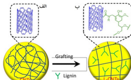
شکل ۴ نانولوله کربنی مربوط به الف) نانولوله‌ی کربنی کلوخه شده، ب) نانولوله‌ی کربنی در پیوند با لیگنین [۵۱].
