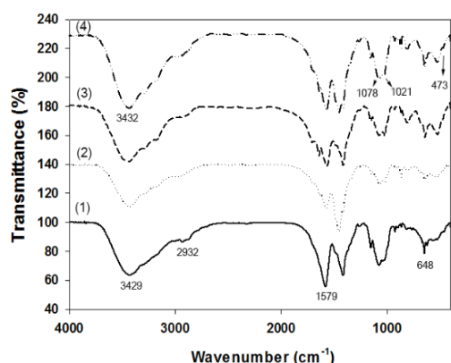
شکل ۵ طیف FTIR مربوط به هیدروژل کیتوزان (Cs) (۱)، Cs&Ph.ZnO@HAP (۲) (۰,۲۵٪)، Cs&Ph.ZnO@HAP (۳) (۰,۵٪) و Cs&Ph.ZnO@HAP (۴) (۱٪).
