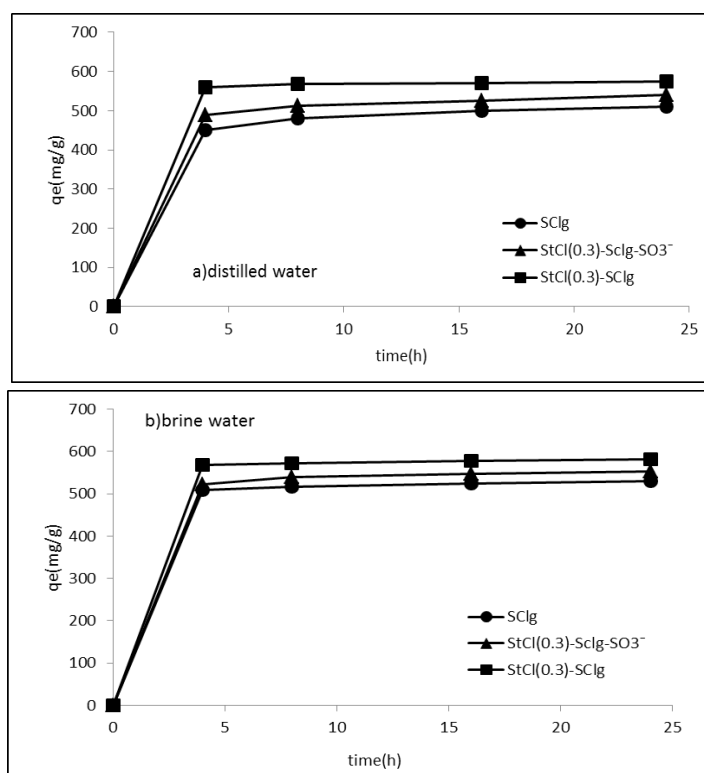
شکل ۵ اثر زمان بر مقدار جذب نمونه اسکروگلوکان اولیه، آب‌گریز و یونی-آب‌گریز در ۲۵ °C (a) محلول آبی، (b) محلول نمکی (غلظت اولیه پلیمر ۰/۳% w/v، غلظت سنگ ۰/۵% w/v)
