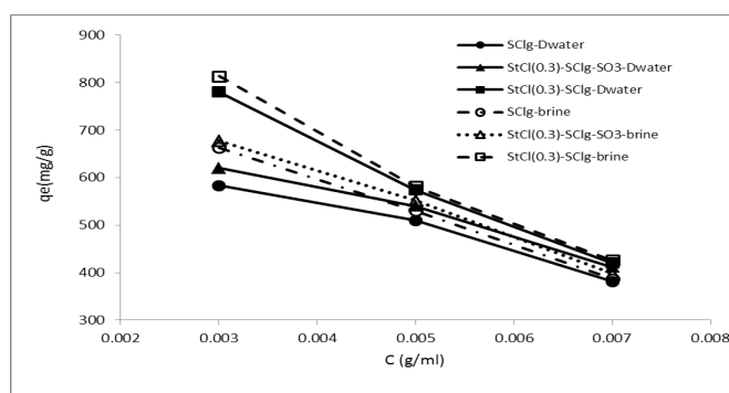
شکل ۶ تأثیر غلظت سنگ مخزن بر مقدار جذب نمونه اسکلوگلوکان اولیه، آب‌گریز و یونی-آب‌گریز در آب مقطر و محلول نمکی (غلظت اولیه پلیمر ۰/۳% w/v، زمان ۲۴ h، دما ۲۵°C)
