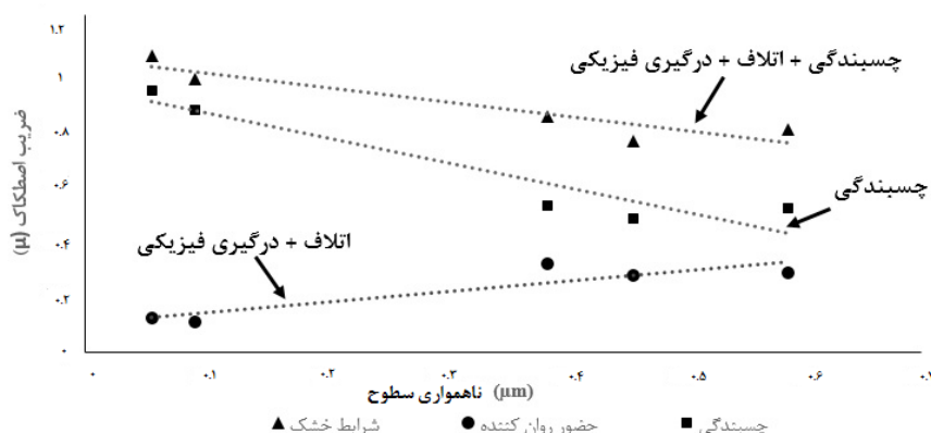
شکل ۹ مقایسه سازوکارهای اصطکاک؛ تغییرات ضریب اصطکاک با ناهمواری سطوح R_a در اصطکاک سُرش
