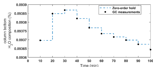
شکل ۴ اندازه‌گیری متغیر PV14 و تخمین آن به کمک سیگنال نگهداری مرتبه صفر
