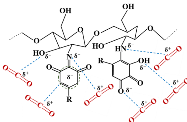
شکل ۹ برهم‌کنش \text{CO}_2 با گروه‌های عاملی لایه گزینش‌پذیر کیتوسان-اسید گالیک Figure 9 Interaction of \text{CO}_2 with functional groups of chitosan-gallic acid selective layer
