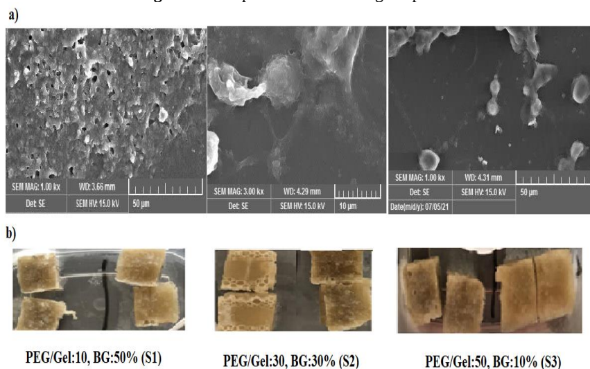
شکل ۷ الف) تصاویر SEM و ب) تصاویر دیجیتالی برای سه داربست S1, S2, S3 Figure 7 a) SEM micrographs and b) digital images for S1, S2, and S3 scaffolds
