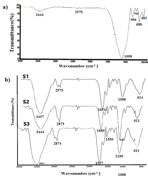
شکل ۵ طیف FTIR مربوط به الف (ب) داربست‌های (S1) PEG/Gel:10, BG:50%, (S2) PEG/Gel:30, BG:30%, و (S3) PEG/Gel:50, BG:10% Figure 5 FTIR spectrum of a) BG and b) scaffolds PEG/Gel:10, BG:50% (S1), PEG/Gel:30, BG:30% (S2), and PEG/Gel:50, BG:10% (S3)
