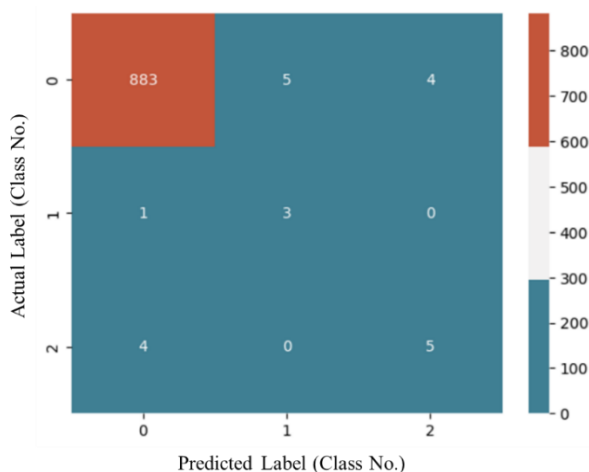
شکل ۷ ماتریس درهم‌ریختگی داده‌های آزمایش با ازای مقدار نگاه به عقب ۵
