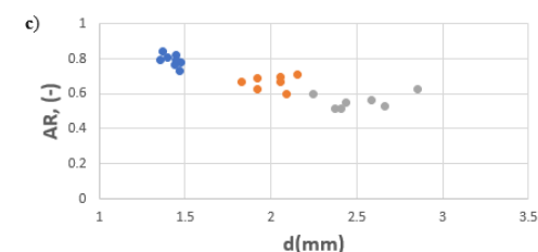
شکل ۷ نسبت ابعادی با اندازه قطرات: (a) در غیاب انتقال جرم، (b) انتقال جرم با غلظت ۲/۴۵ میلی‌مولار و (c) انتقال جرم با غلظت ۲۴/۵ میلی‌مولار
