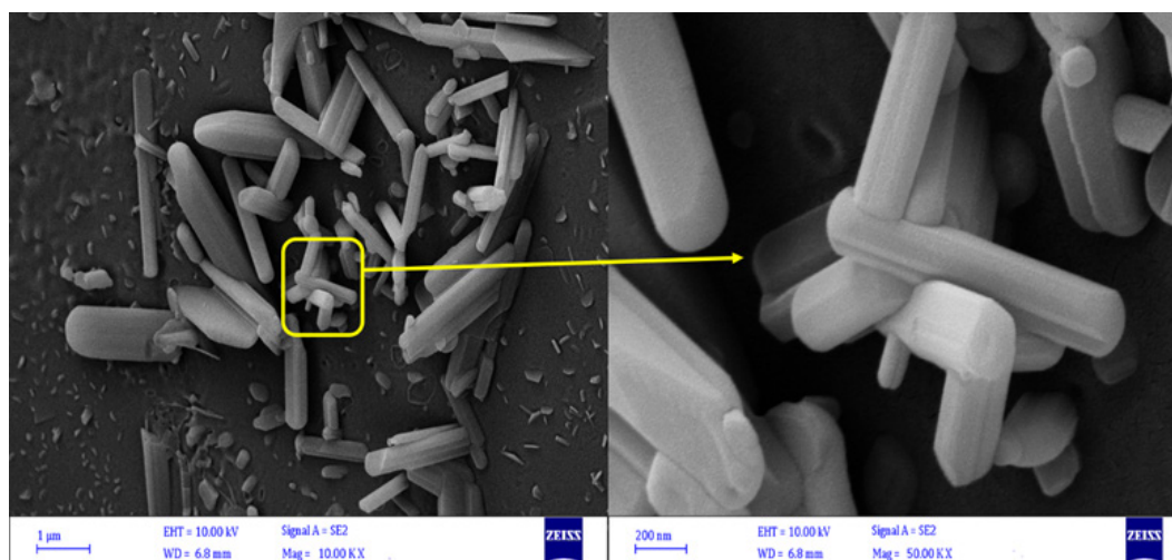
شکل ۴ تصویر FESEM کاتالیزور سنتز شده V/PERLIT-IA(۱،۵) Fig. 4 FE-SEM images of the synthesized V/PERLIT-IA(1.5) catalyst
