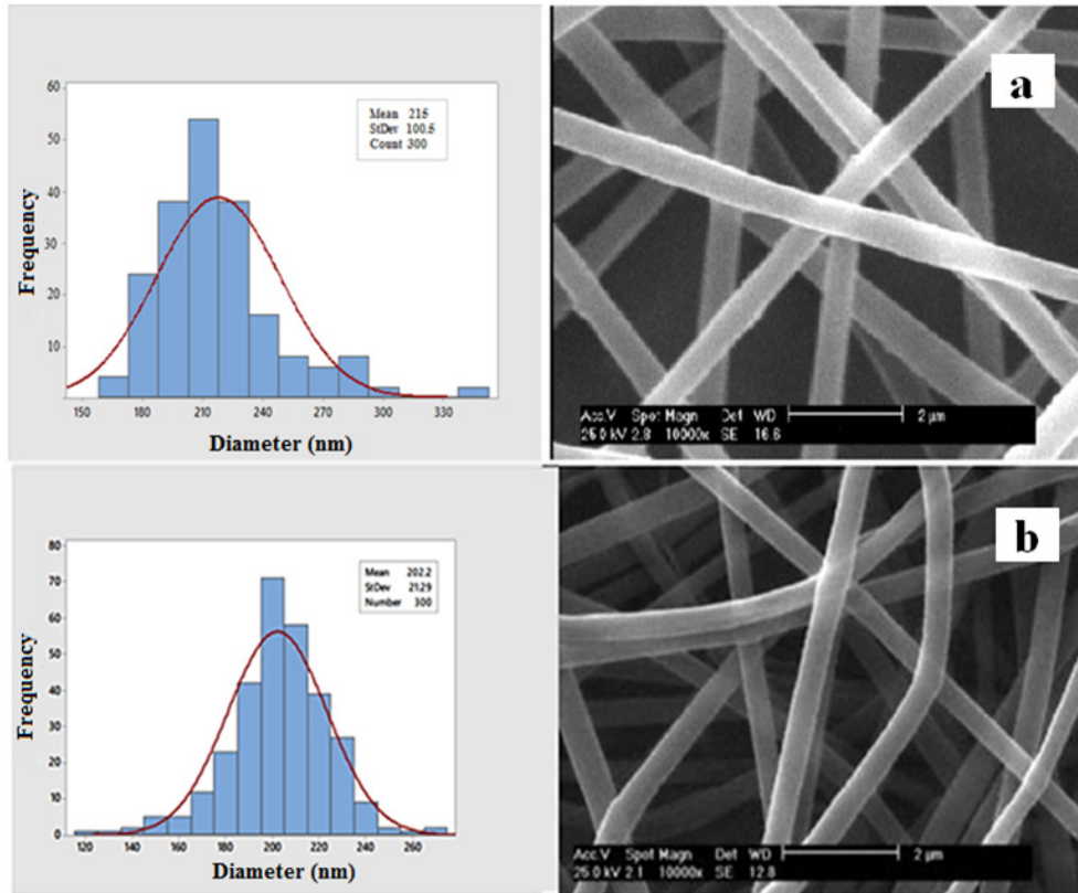
شکل ۲ تصاویر SEM و توزیع قطر نانو الیاف با شرایط بهینه الکترورسی. الف) پلی‌آمید ۶ با غلظت wt. ۱۵٪، نرخ تغذیه ۰/۵ ml/h، ولتاژ ۲۰ kV و فاصله ۱۰ cm، و ب) پلی وینیل الکل با غلظت wt. ۸٪، نرخ تغذیه ۰/۲ ml/h، ولتاژ ۲۰ kV و فاصله ۱۵ cm.
