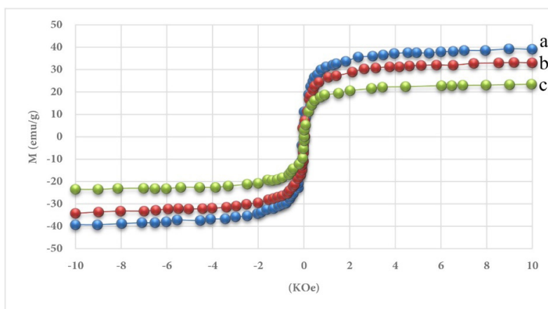
شکل ۴ منحنی مغناطیسی برای (a) \text{MnFe}_2\text{O}_4 ، (b) \text{TiO}_2\text{-MnFe}_2\text{O}_4 و (c) \text{UIO-66-MnFe}_2\text{O}_4\text{-TiO}_2 Figure 4 Magnetic curve for (a) \text{MnFe}_2\text{O}_4 , (b) \text{TiO}_2\text{-MnFe}_2\text{O}_4 and (c) \text{UIO-66-MnFe}_2\text{O}_4\text{-TiO}_2
