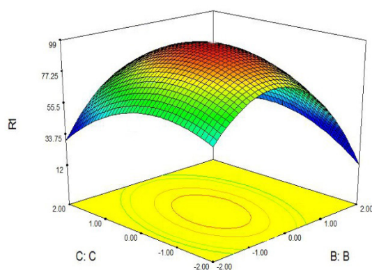
شکل ۱۰ تأثیر زمان جذب (C:C) و pH (B:B) بر روی جذب \text{Cr(VI)} به وسیله جاذب سنتز شده Figure 10 Effect of adsorption time (C: C) and pH (B:B) on the adsorption of Cr (VI) by the synthesized adsorbent
