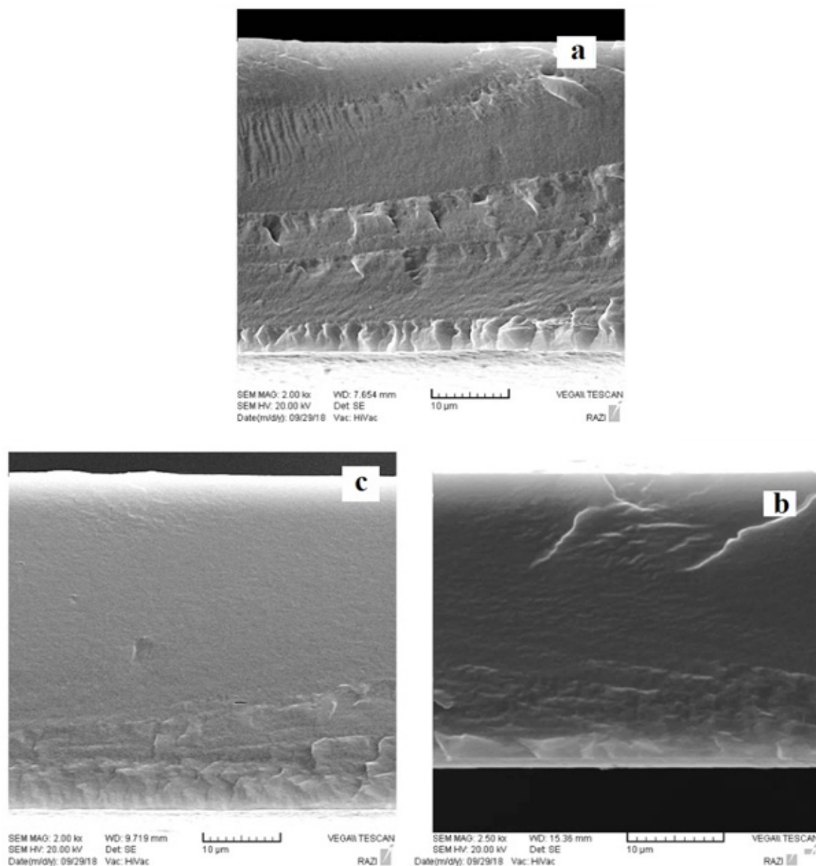
شکل ۱- تاثیر افزودن PEG به شبکه پلیمر Pebax (a) غشا خالص Pebax ® 1657 ، (b) غشا حاوی ۵٪ وزنی PEG (c) غشا حاوی ۱۰٪ وزنی PEG Figure 1. Effect of adding PEG into Pebax matrix (a) pure Pebax ® 1657 (b) membrane contains %5wt PEG (c) membrane contains %10wt PEG
