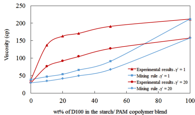
شکل ۱۳: تأثیر نرخ برش بر سازگاری نمونه‌ها قبل از پیرسازی در آب شیر (دمای ۲۵°C، نرخ برش‌های ۱/s و ۲۰/s) Figure 13 Effect of shear rate on the compatibility of the blend components before aging at tap water (at 25°C)
