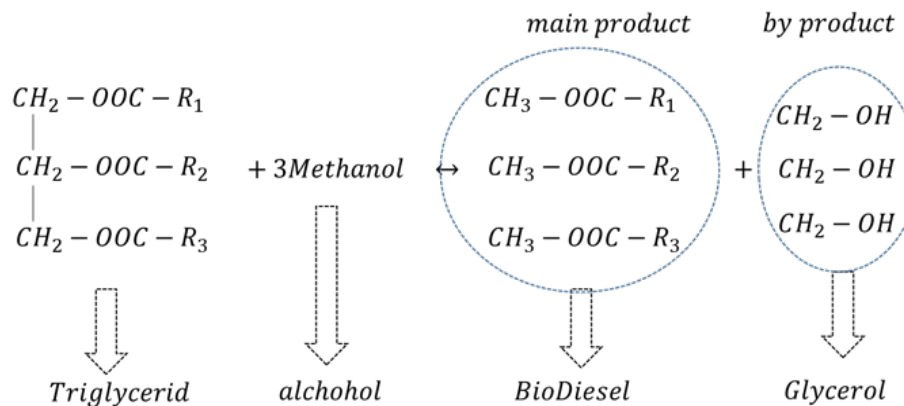
شکل ۱ واکنش استری شدن تبادل و تولید بیودیزل و گلیسرین [۱۷] Fig. 1. Transesterification reaction and production of biofuels and glycerin [17]
