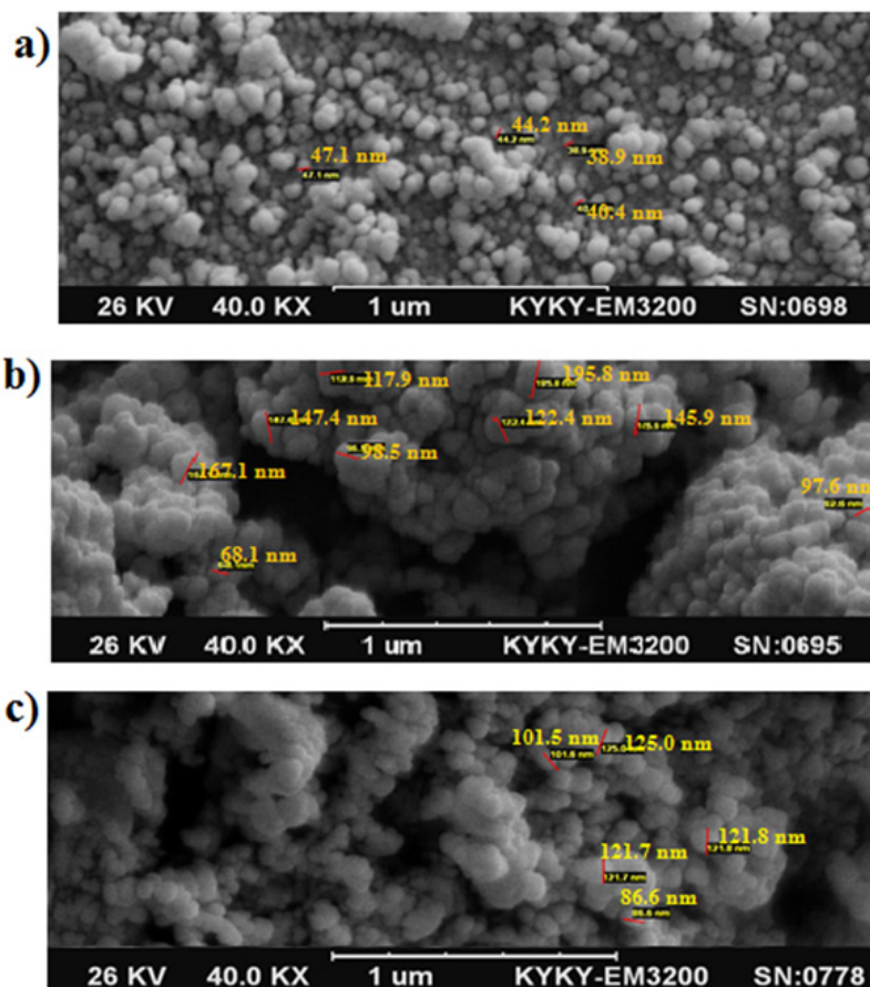
شکل ۷ تصاویر SEM از نانوذرات (a) ZnO، (b) نانوکامپوزیت ZnO / Chitosan، (c) نانوکامپوزیت ZnO / Chitosan / Metformin Figure 7. SEM images of the (a) ZnO nanoparticles, (b) ZnO/Chitosan, (c) ZnO/Chitosan/Metformin nanocomposite
