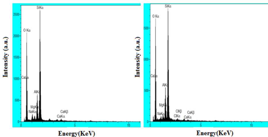
شکل شماره ۳. آنالیز عنصری بنتونیت خام (چپ) و بنتونیت اصلاح شده با روش اسیدی- گرمایی (راست)
